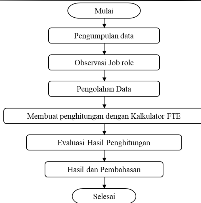
Gambar 2.3 . Langkah Penelitian
